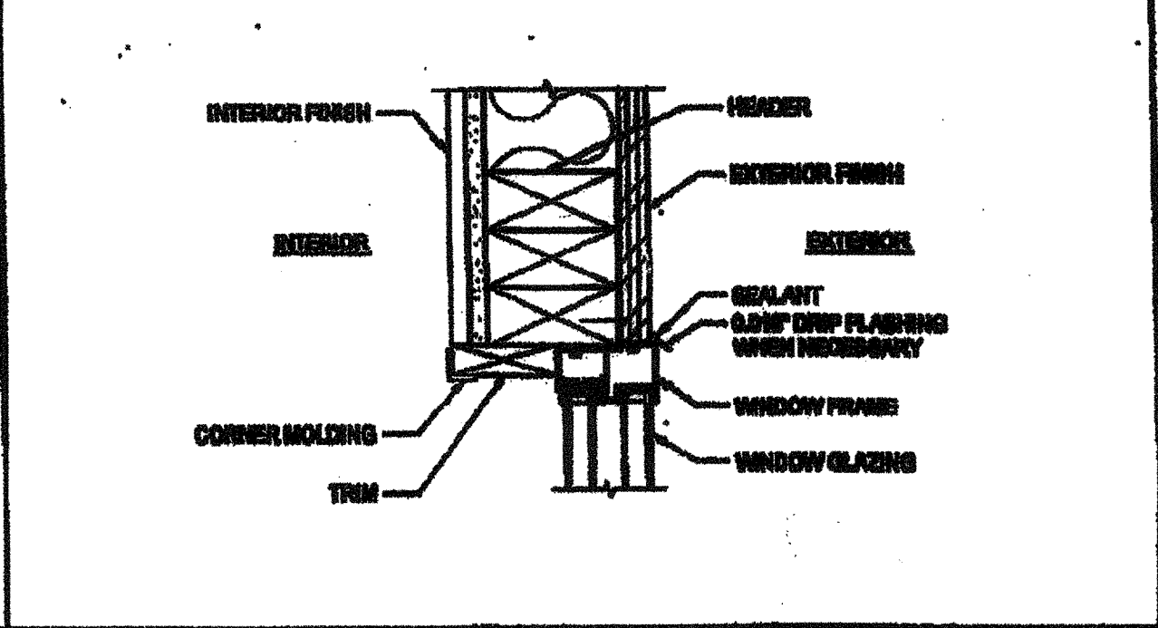
WINDOW HEADER SCALE: 3/4"=1'-0" 12
