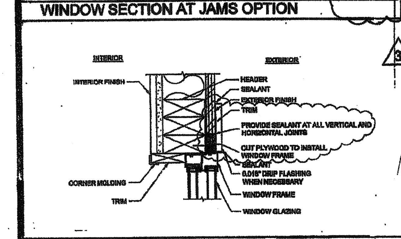
WINDOW HEADER - OPTION SCALE: 3/4"=1'-0" 20
